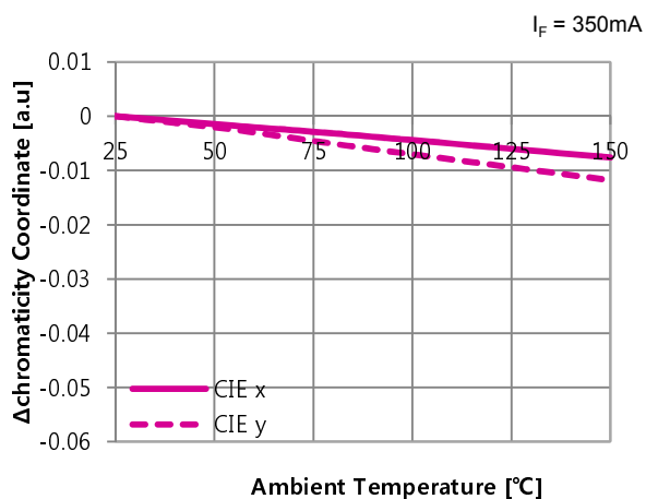
▪ CIE vs. Ambient Temp.
