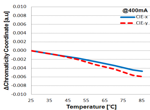
■ CIE vs. Temp.
