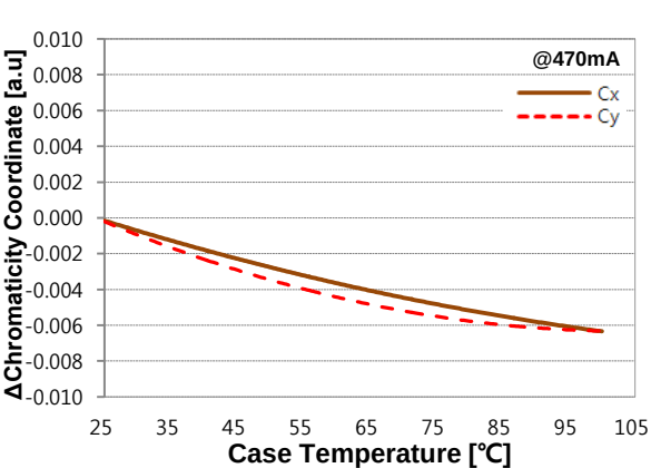
■ CIE vs. Temp.
